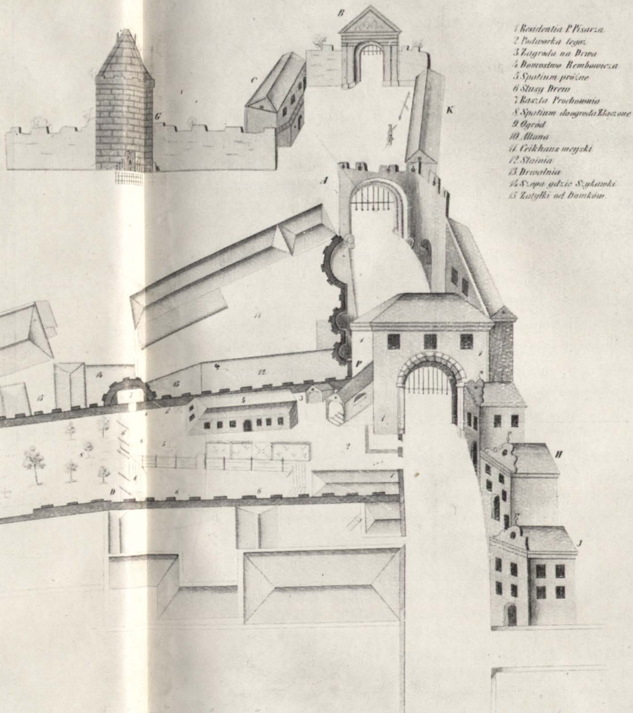
Plan bram Nowomiejskich. (Wejnert, Star. Warsz. T. I.).
